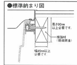
標準型の納まり図
