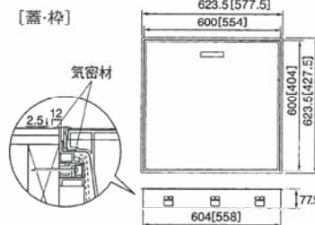
〔蓋・枠〕
