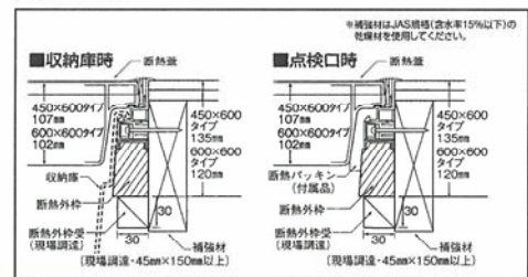
断熱型の納まり図
