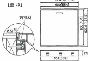
〔蓋・枠〕
