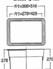
製品寸法
