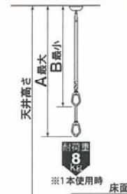
基本納まり寸法図
