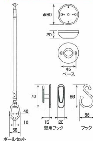
部品寸法図
