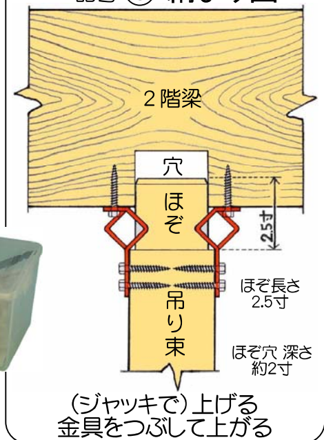
記号 ㊧ 納まり図
