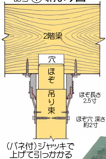
記号 ㊦ 納まり図
