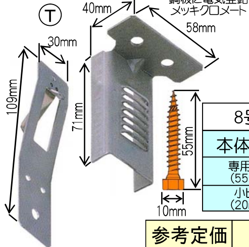
かもい上げ金具
